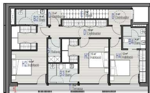
3 Planta Primera
