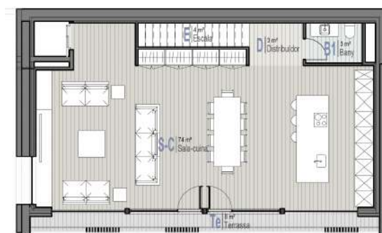
4 Planta Segona
