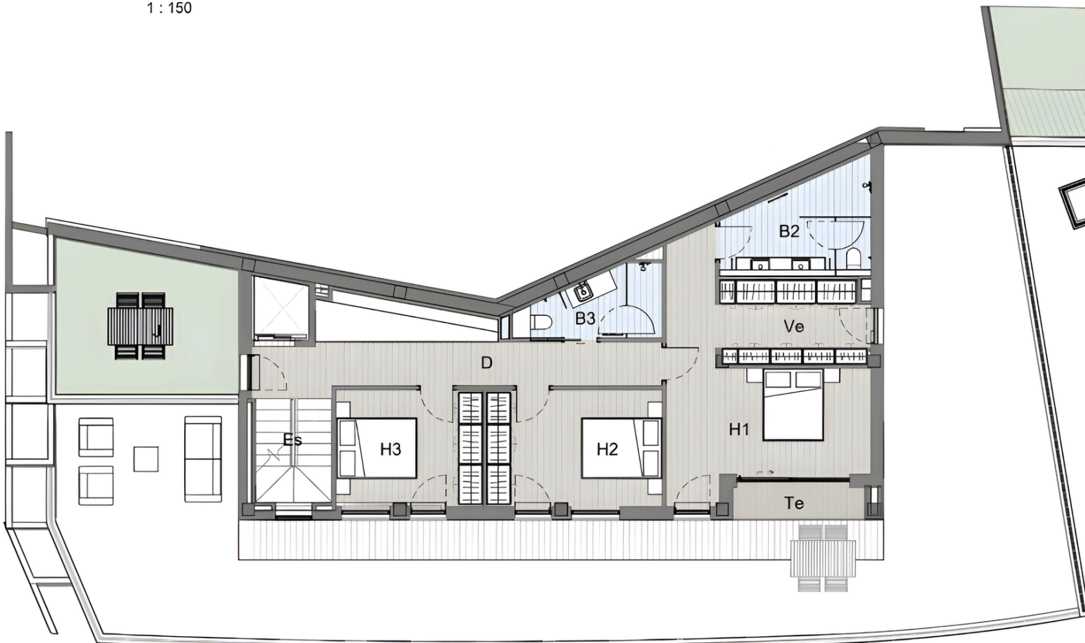
1 Xalet 2 - P-1 - Venda 1 : 150
