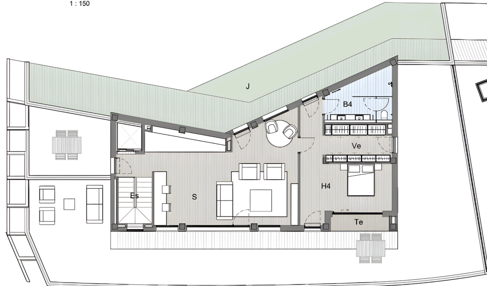
2 Xalet 2 - PB - Venda 1 : 150
